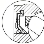
密封型式2RS Seal Type 2RS
